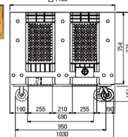
< 기본형 캐스터 부착시 / 전면 >
